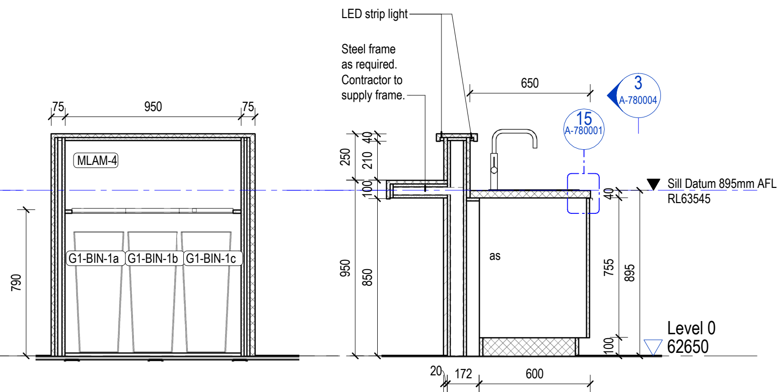
4 JO-BW-1 Section 1 1 : 20
