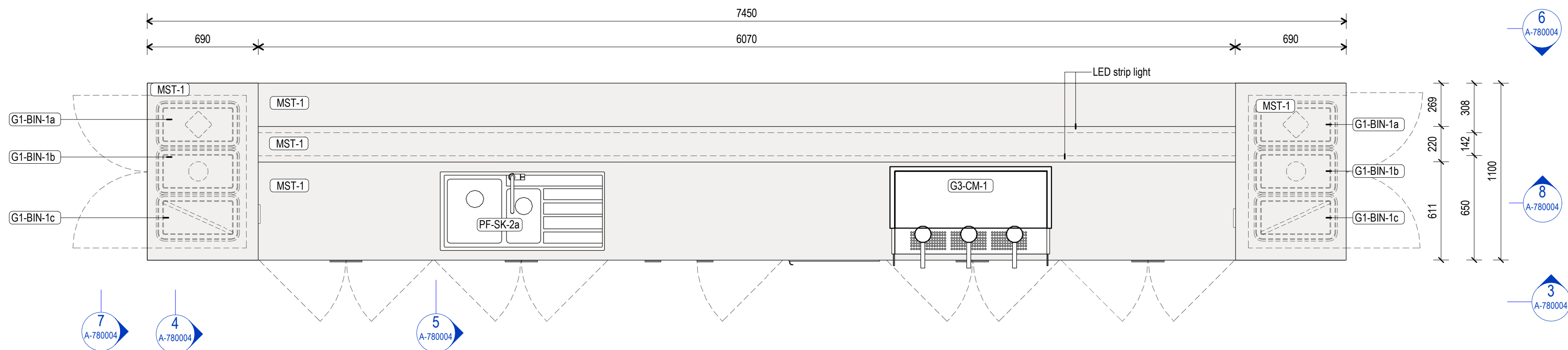
2 JO-BW-1 Plan 1 : 20
