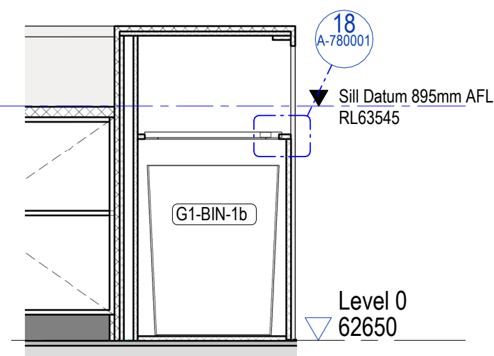
8 JO-BW-1 Section 3 1 : 20
